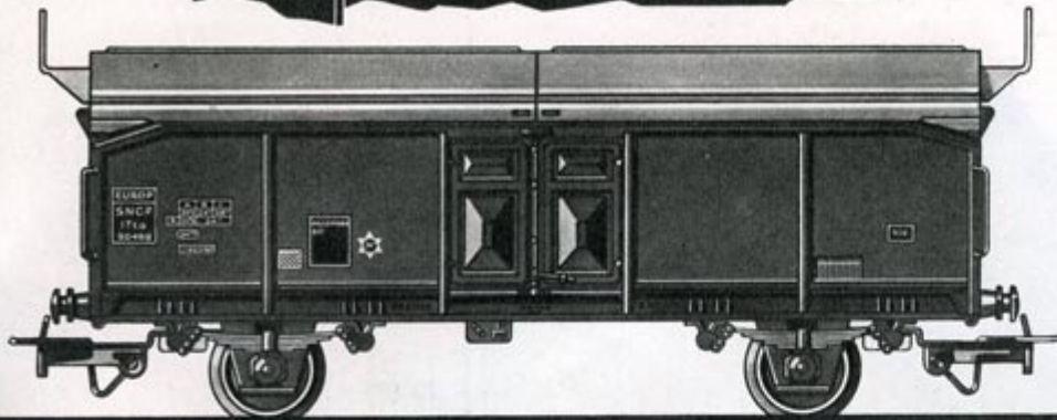
Tondereau à toit coulissant. Réf. 622. ITto. S.N.C.F. Licence S.E.A.G. Longueur du châssis 107 mm.
