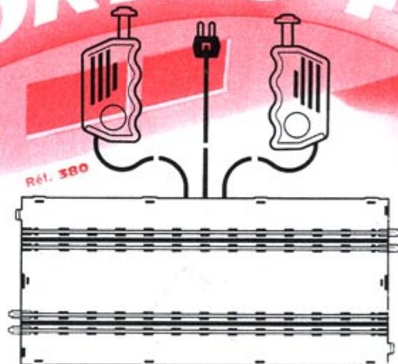
Route « alimentation ». Réf. 310 A. Longueur : 260 mm.
