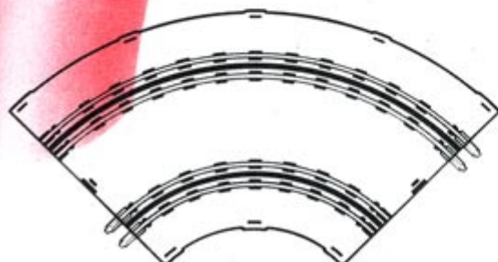
Route courbe : 90°. Réf. 320. Rayon moyen : 130 mm. 1/2 Route courbe : 45°. Réf. 320/2. Rayon moyen : 130 mm.
